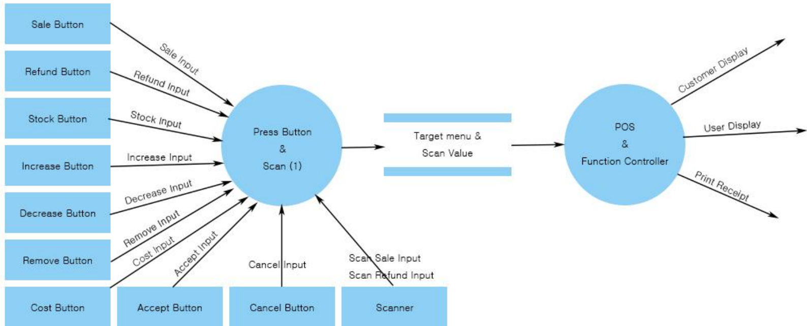
DFD Level 1
